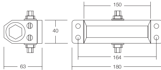
Diagram G 80 / G 801 / G 801BC / G 802H
